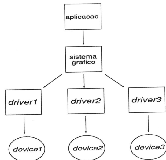
Figura 2: aplicações gráficas com sistemas gráficos.
