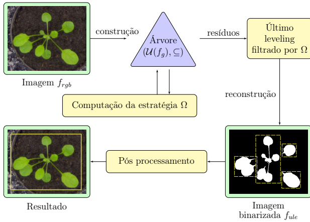
Figura 3. Visão geral da nossa abordagem para a tarefa de detecção do bounding box da planta. Note que, a imagem f_{rgb} é apenas um recorte.
