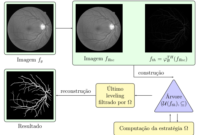
Figura 4. Visão geral da nossa abordagem para a aplicação de segmentação de vasos sanguíneos em imagens de retina.
