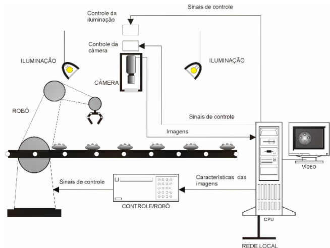
Figura 3. Linha de produção manufaturada com inspeção automatizada por meio de um sistema de visão de máquina [7].
