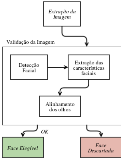
Figura 3. Fluxograma da etapa de extração e processamento de imagens.
