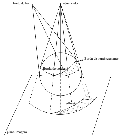
Figura 5: Borda de oclusão para observador e fonte de luz em posições diferentes
