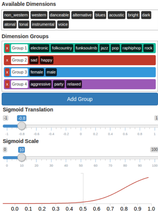
Fig. 4. Application menu.
